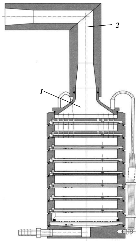
Рис. 2 – Каскадный импактор Андерсена в конфигурации для анализа аэрозолей
