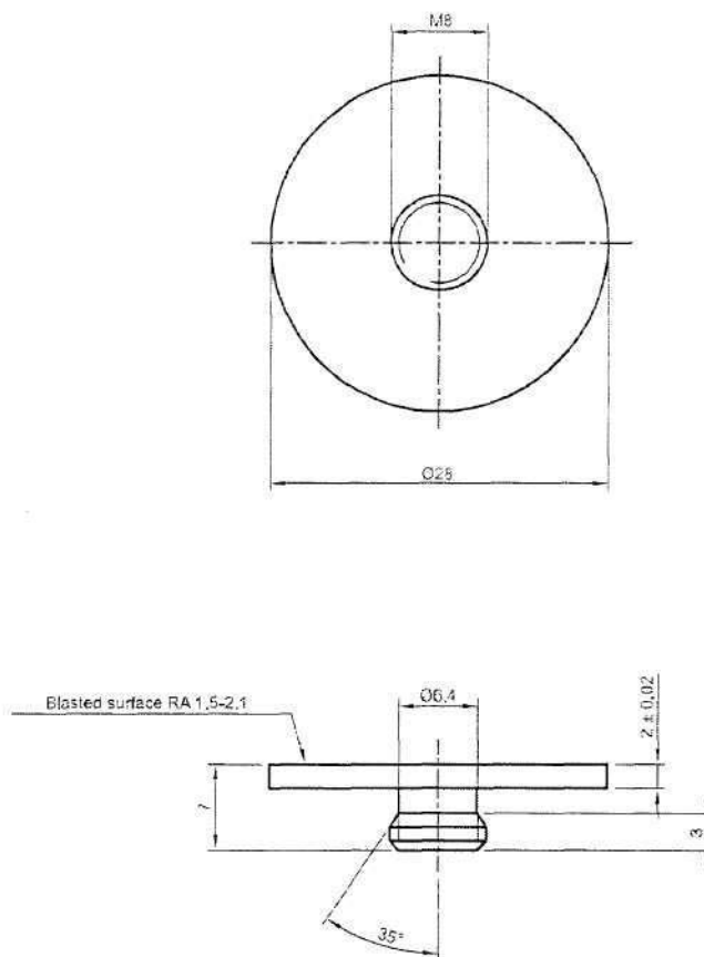
Рисунок 9 – Прибор Б. Верхняя поверхность имитации жевания Размеры указаны в мм
