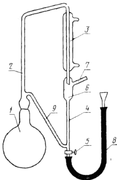
Рис. 2 – Прибор для определения эфирного масла методами 2 и 3
