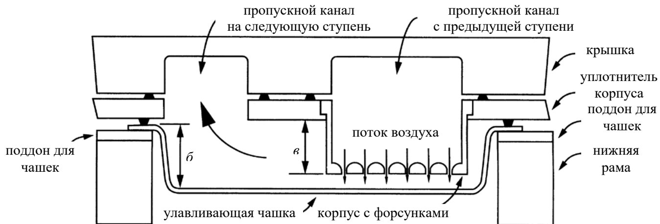
Рис. 11 – Схема межступенчатых каналов каскадного импактора нового поколения
