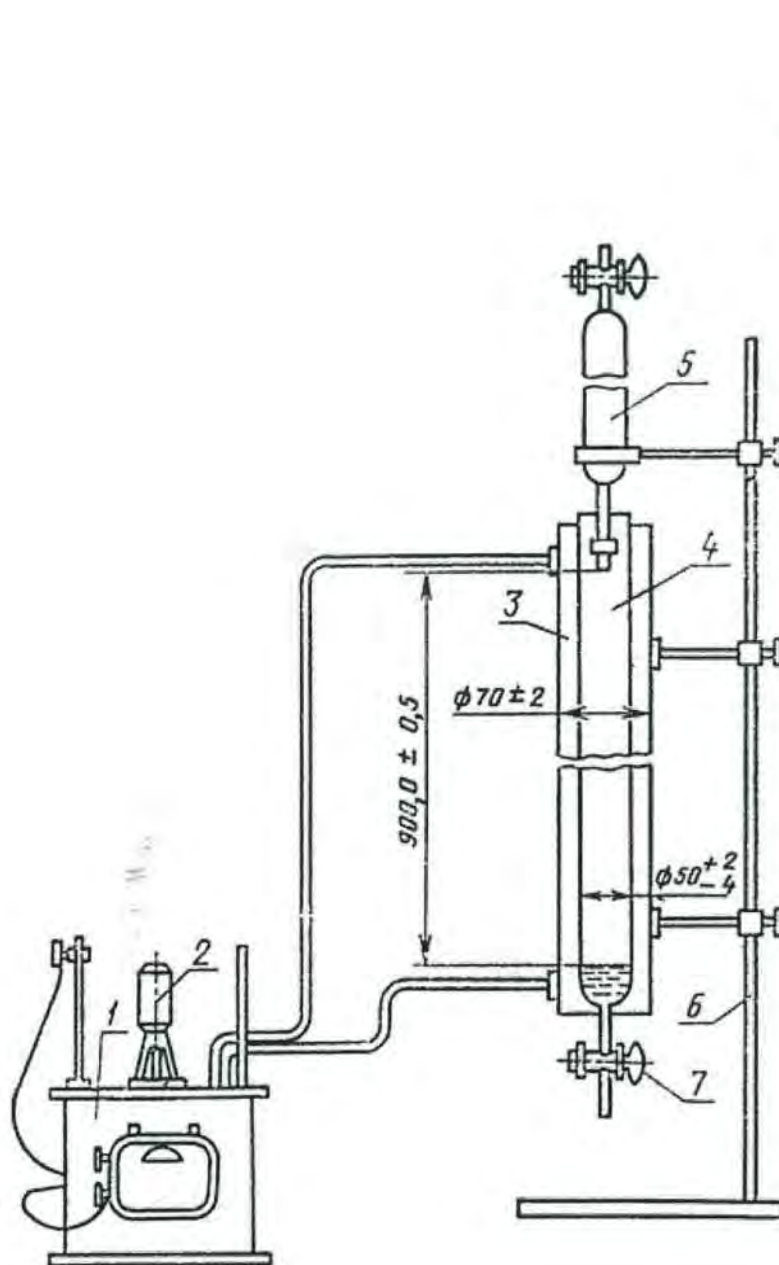
Рис. 1 – Прибор Росс-Майлса 1- термостат, 2- насос, 3-водяная рубашка, 4-мерный цилиндр, 5- стеклянная пипетка, 6-штатив Размеры указаны в мм
