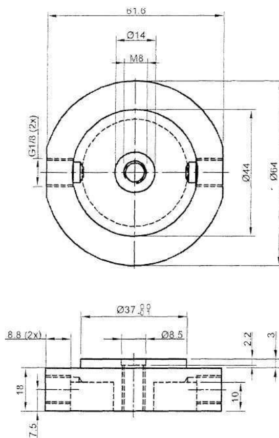
Рисунок 8 – Прибор Б. Камера-основание Размеры указаны в мм
