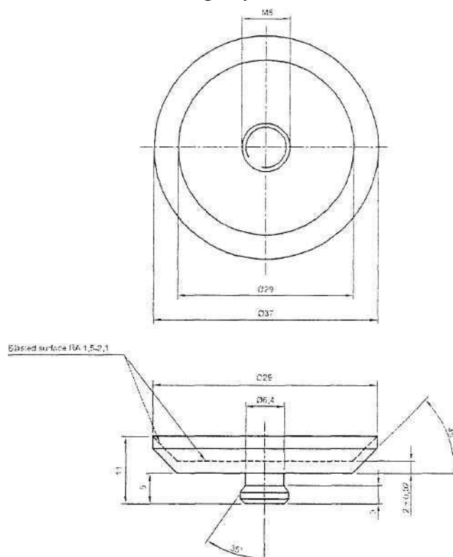
Рисунок 10 – Прибор Б. Нижняя поверхность имитации жевания Размеры указаны в мм
