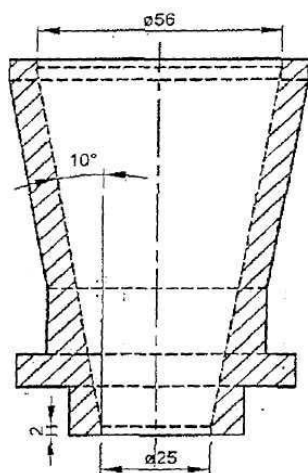
Рисунок 2 – Прибор А. Воронка Размеры указаны в мм
