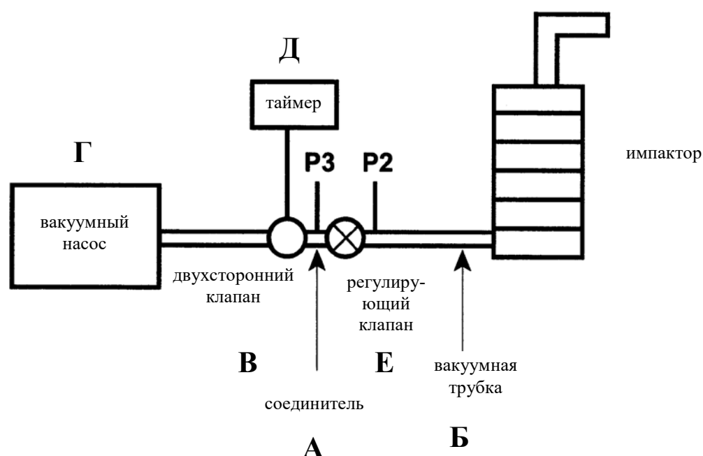
Рис. 4 – Система регулирования воздушного потока
