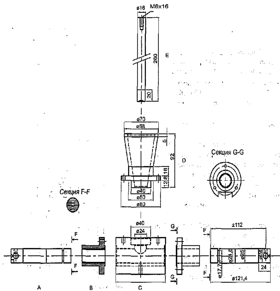
Рисунок 1 – Прибор А для имитации жевания.
