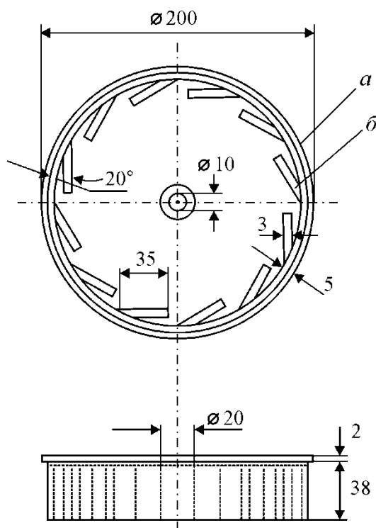
Рис. 1 – Прибор для определения истираемости таблеток
