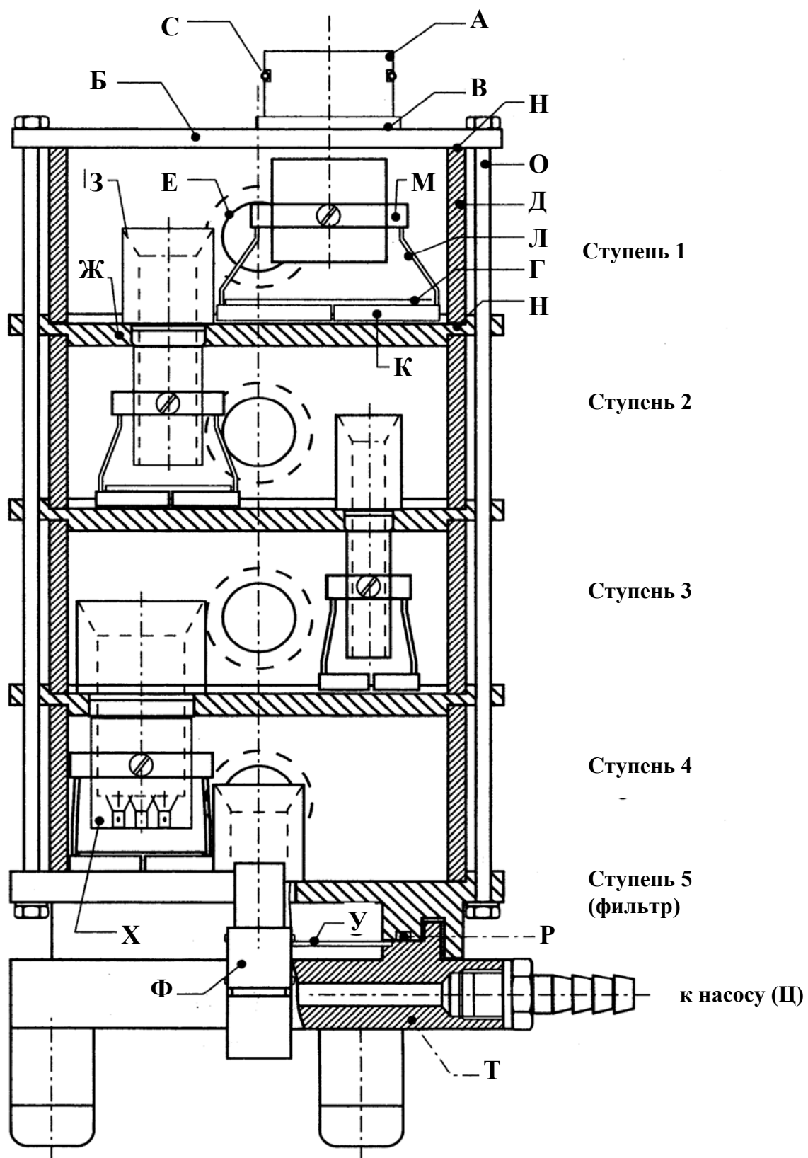
Рис. 5 – Многоуровневый жидкостной импиджер
