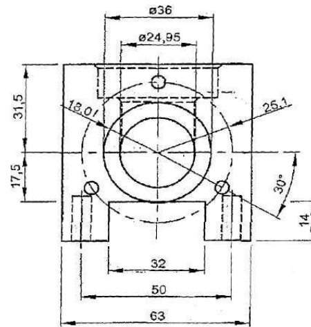
Рисунок 3 – Прибор А. Направляющая Размеры указаны в мм
