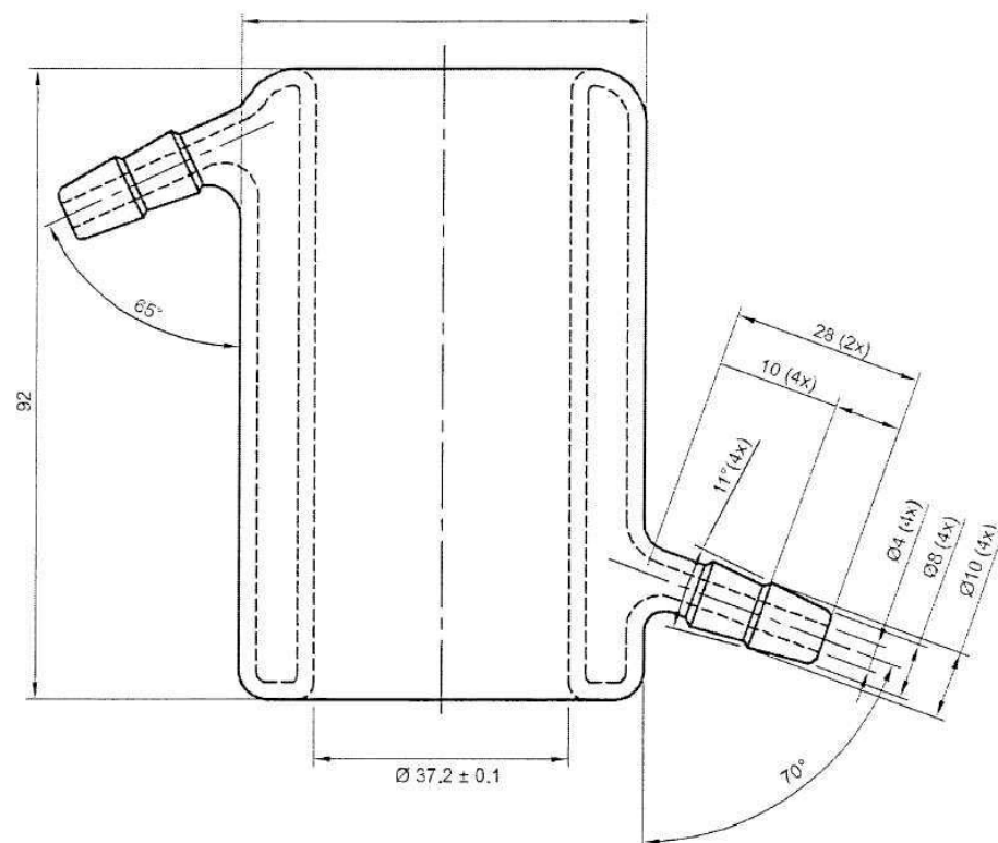
Рисунок 5 – Прибор Б. Ячейка для испытания Размеры указаны в мм
