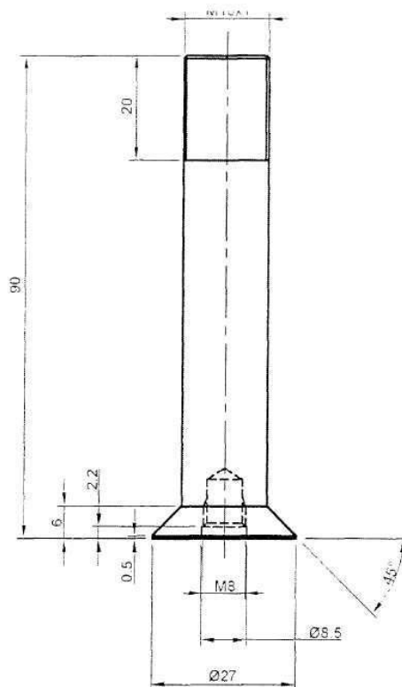
Рисунок 7 – Прибор Б. Шток Размеры указаны в мм
