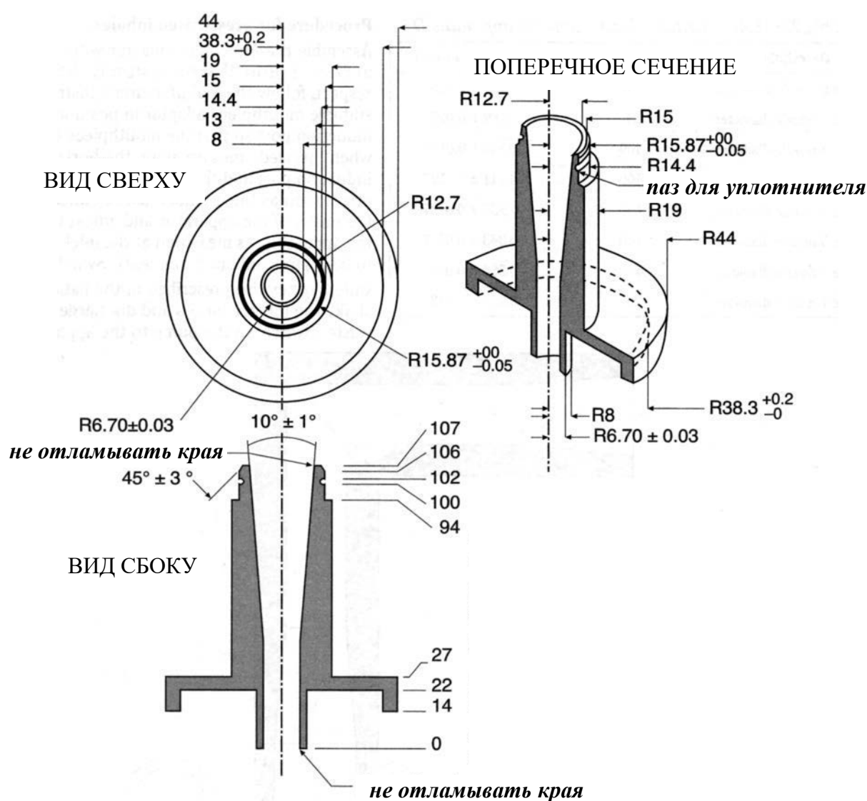
Рис. 3 – Пресепаратор для каскадного импактора Андерсена
