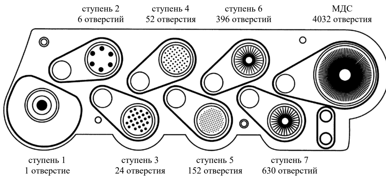
Рис. 12 – Конфигурация форсунок импактора нового поколения
