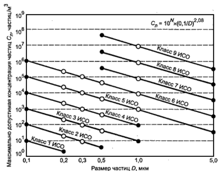
Рисунок А.1 - Графическое представление границ классов ИСО
